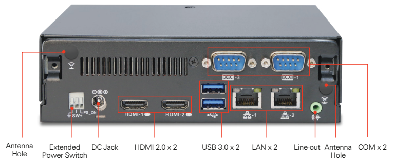
COM x 2
